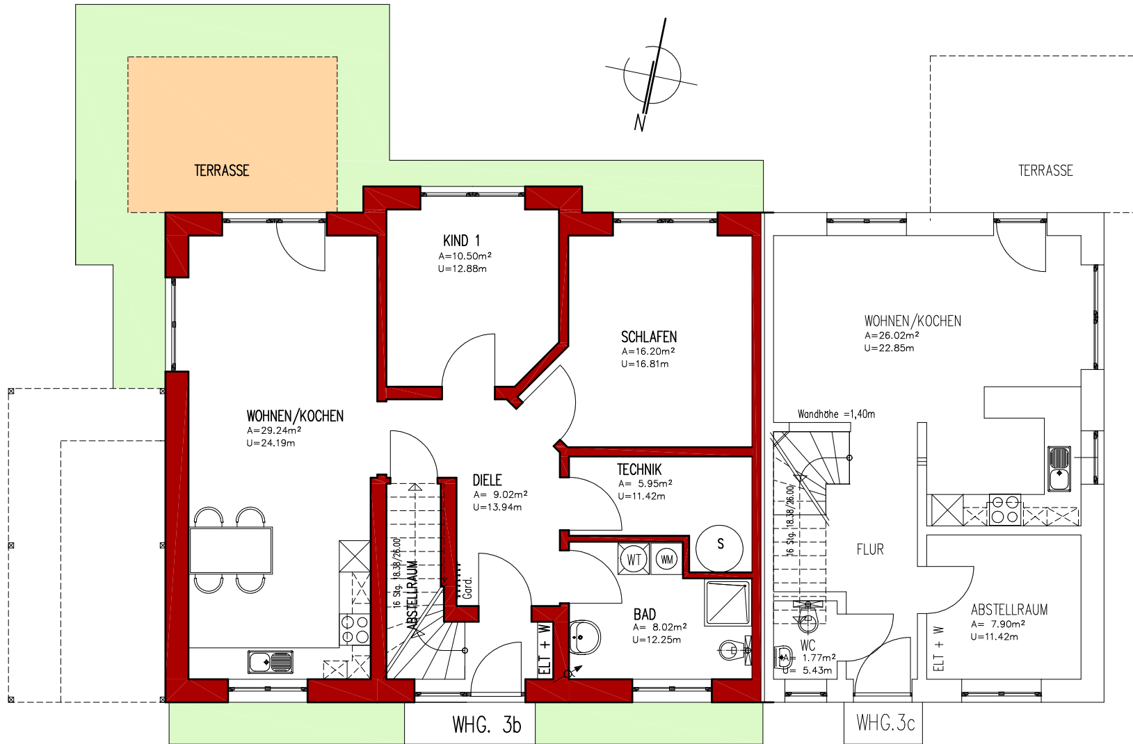
ERDGESCHOSS
