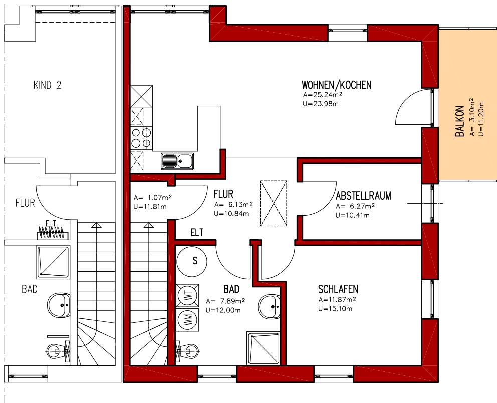
OBERGESCHOSS EINLIEGERWOHNUNG
